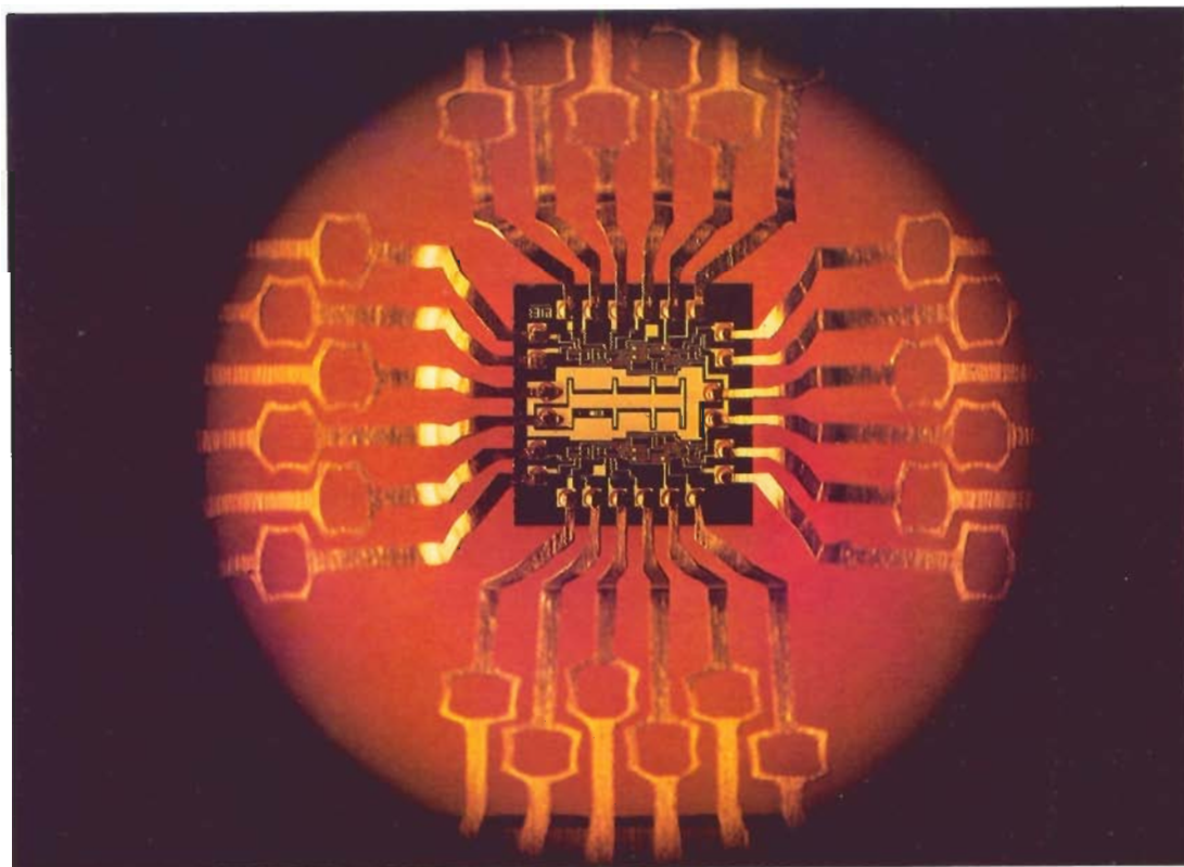
Premier niveau d'interconnexion d'une puce par la technique du T.A.B. (Tape Automatic Bonding) (Bull).
